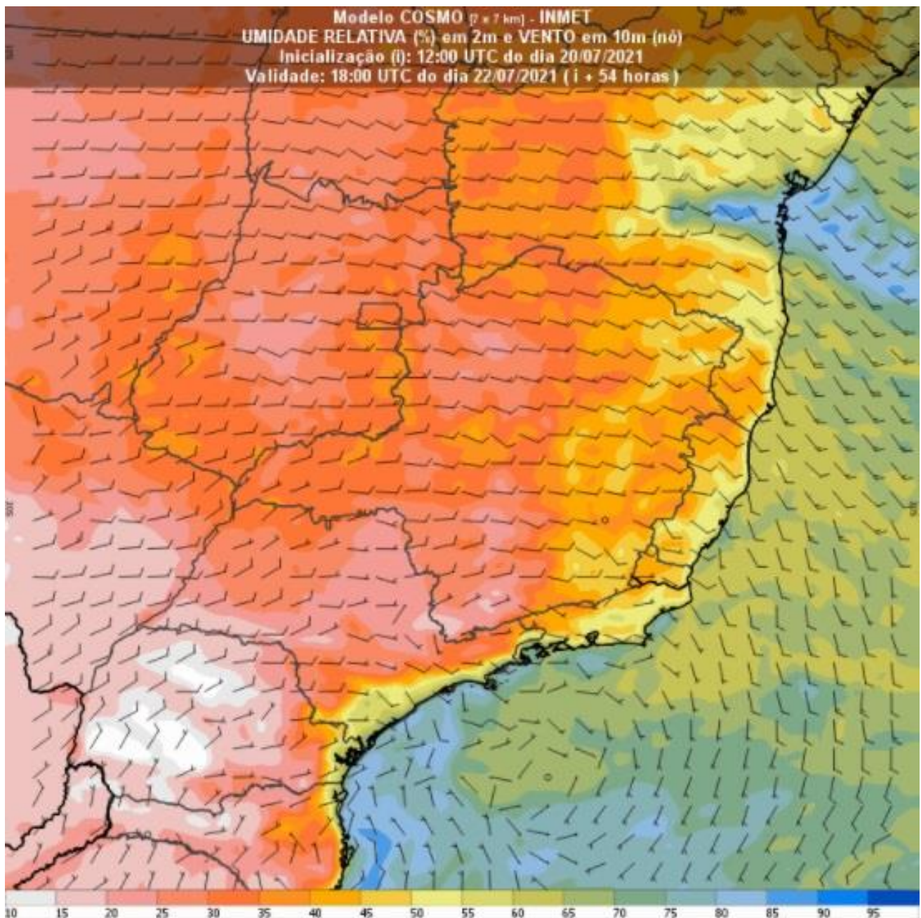
Figura 1 – Simulação do modelo COSMO/INMET com a Umidade Relativa do Ar.
