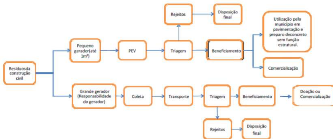
Figura 5.5 – Fluxograma do manejo adequado dos resíduos da construção civil
