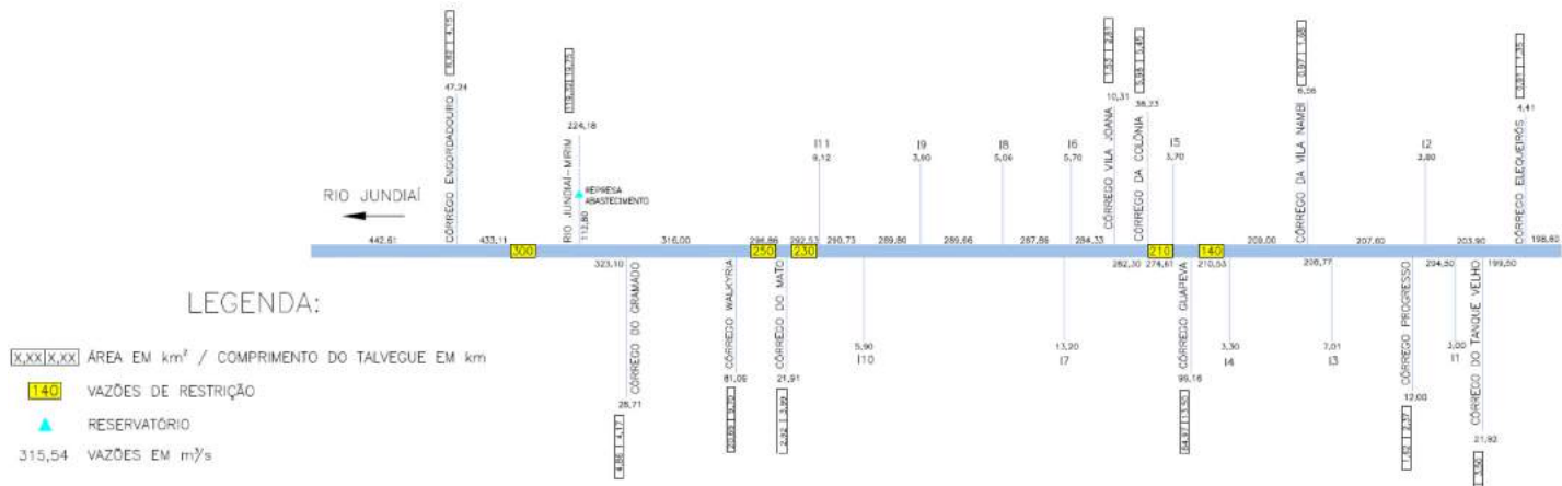
Figura 5.2 - Prognóstico da Macrodrenagem – TR – 25 anos – condição futura de ocupação
