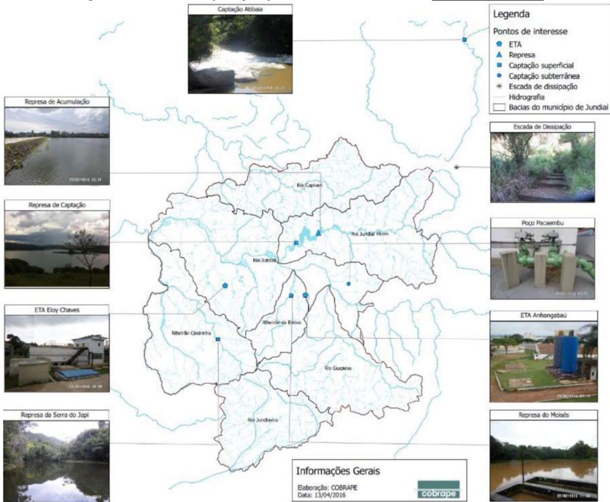
Figura 4.2 - SAA em operação pela DAE S.A. em Jundiaí ETA-Anhangabaú
