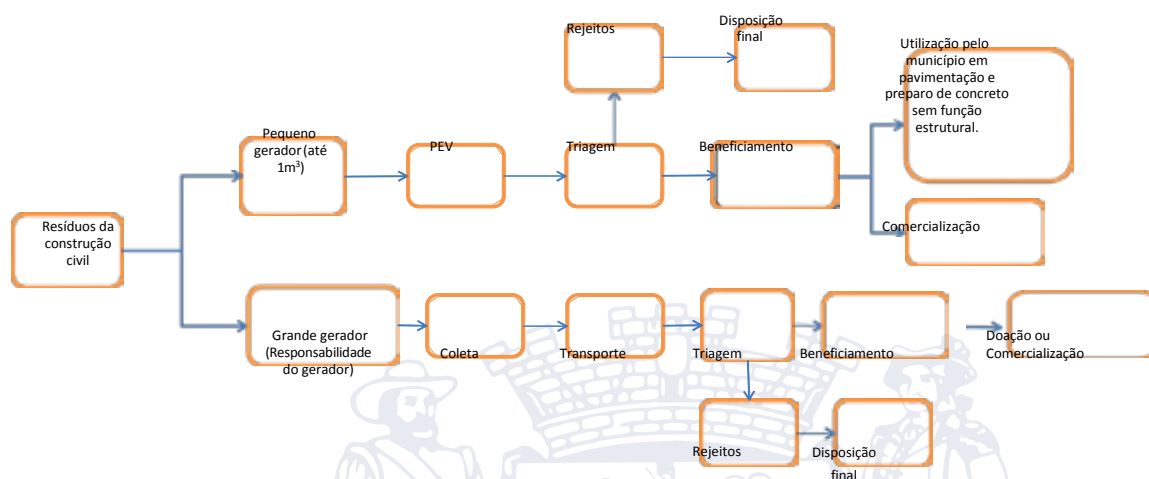
Figura 22: Fluxograma do manejo adequado dos resíduos da construção civil.
