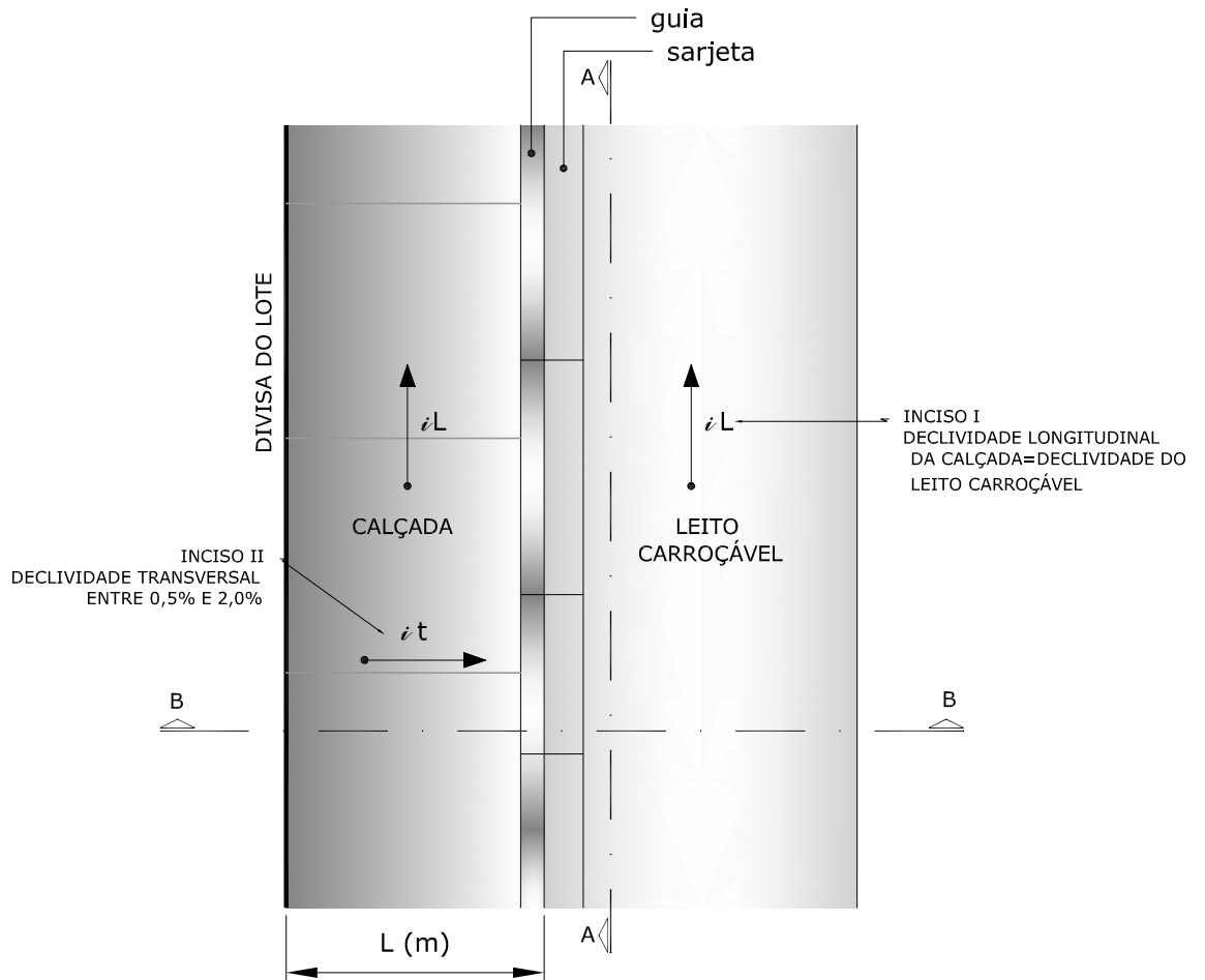
VISTA EM PLANTA
