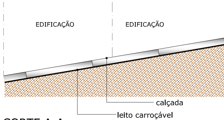
VISTA CORTE A-A
