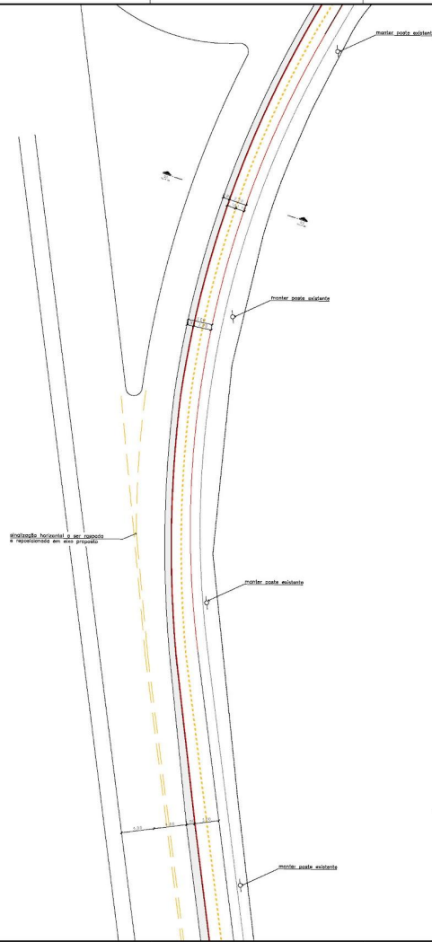
TRECHO 03 ESCALA 1:200
