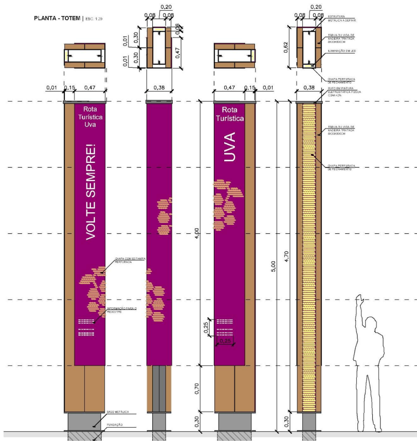
ELEVAÇÕES - TOTENS | ESC: 1:20
