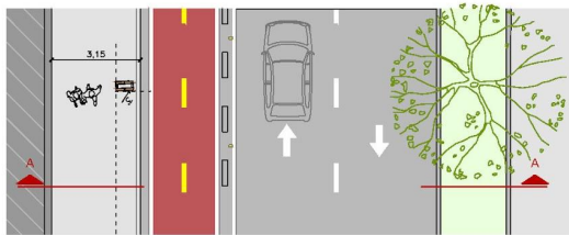
IMPLANTAÇÃO | ESC: 1:100
