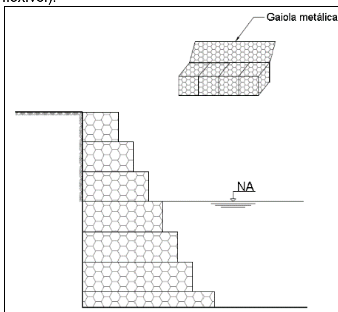
Figura 51 – Revestimento de gabião (revestimento flexível).
