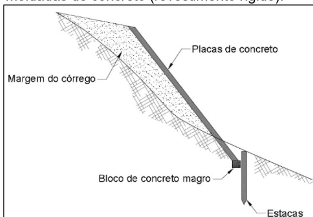
Figura 52 – Revestimento com placas pré-moldadas de concreto (revestimento rígido).
