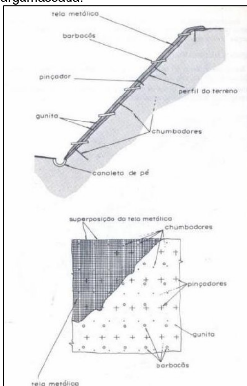
Figura 37 – Proteção superficial com tela argamassada.
