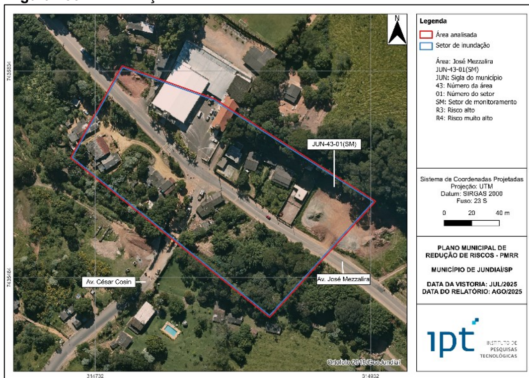
Figura 136 – Delimitação dos setores de risco.
