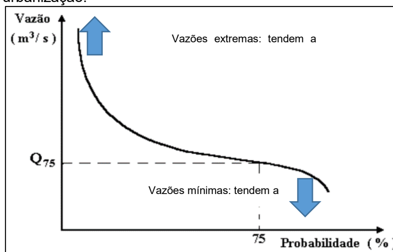
Figura 30 – Curva de permanência de vazões. Impactos da urbanização.
