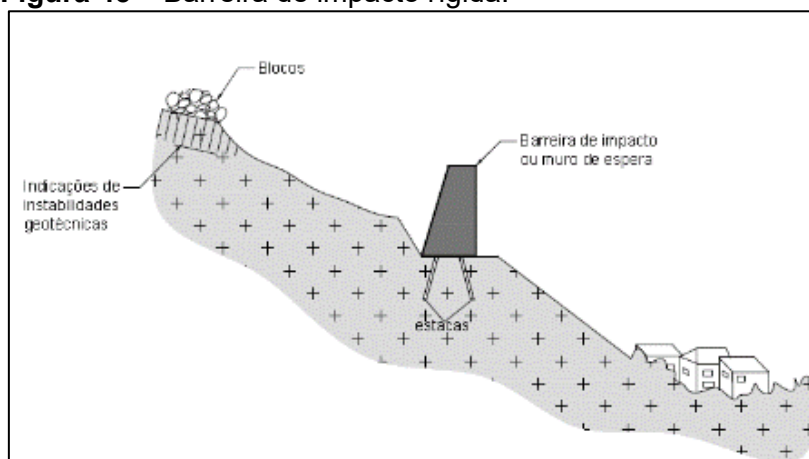
Figura 45 – Barreira de impacto rígida.
