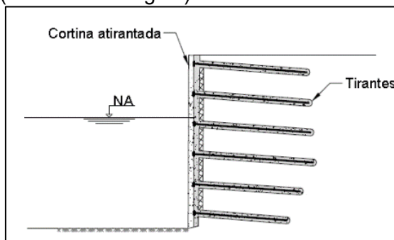
Figura 53 – Cortina atirantada (revestimento rígido).
