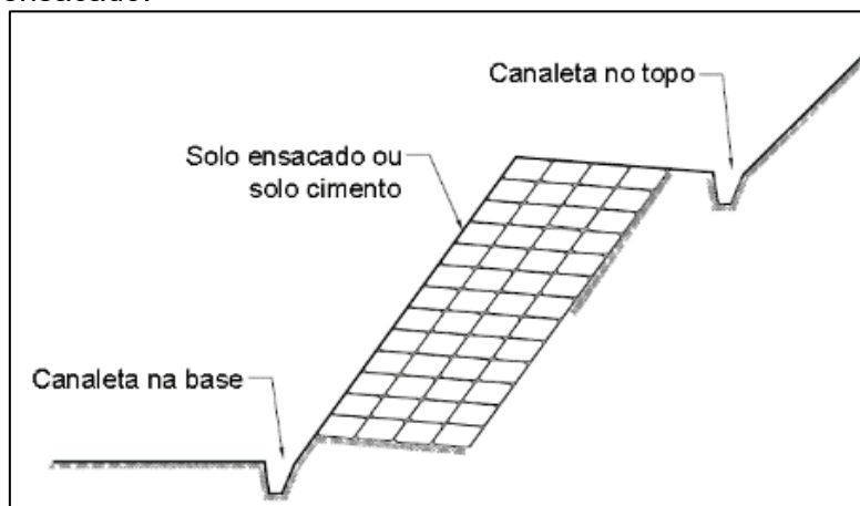
Figura 44 – Contenção com muros de saco-cimento ou solo ensacado.
