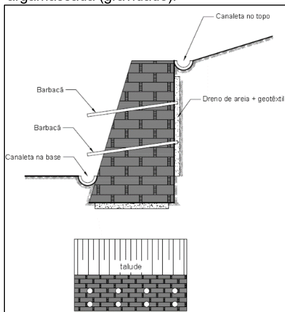
Figura 40 – Contenção com muro de pedra argamassada (gravidade).
