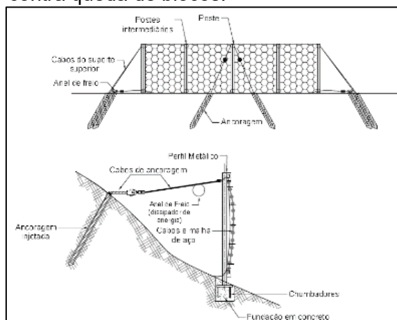
Figura 46 – Barreira de impacto flexível contra queda de blocos.
