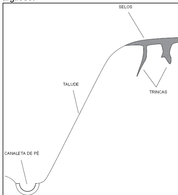
Figura 34 – Proteção com selos de solo argiloso.
