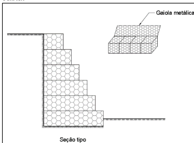
Figura 41 – Contenção com muro de gabião-caixa.
