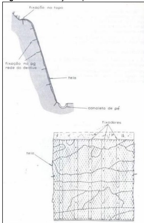
Figura 38 – Proteção superficial com tela.
