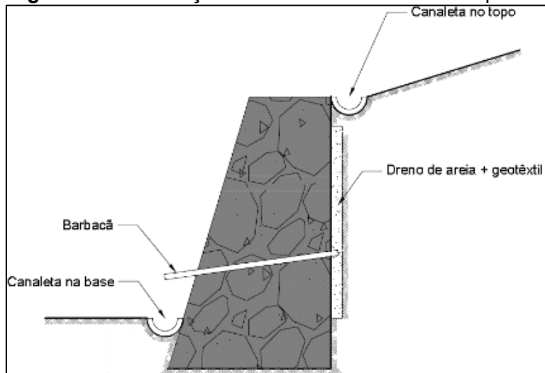
Figura 42 – Contenção com muro de concreto ciclópico.
