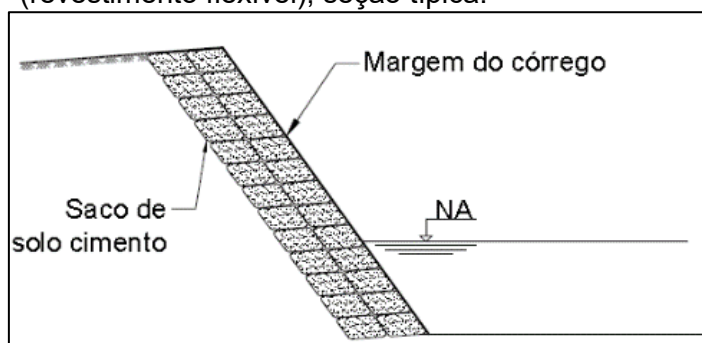
Figura 50 – Revestimento com enrocamento sintético (revestimento flexível); seção típica.
