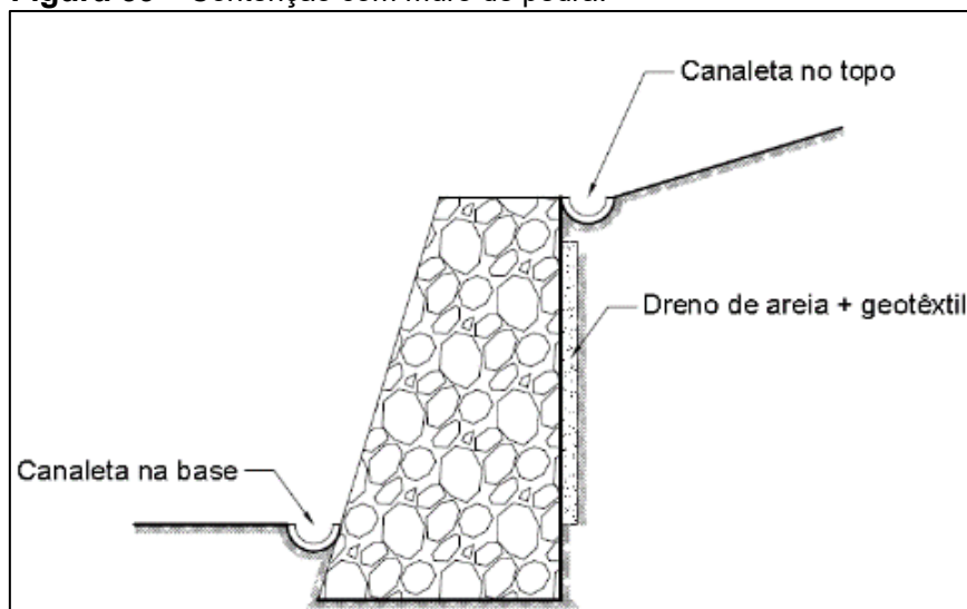
Figura 39 – Contenção com muro de pedra.
