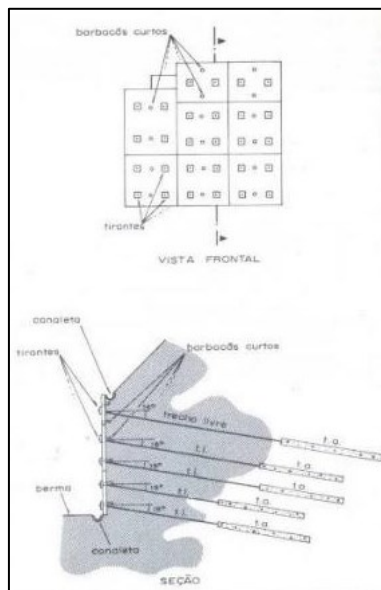
Figura 49 – Contenção com cortina atirantada.
