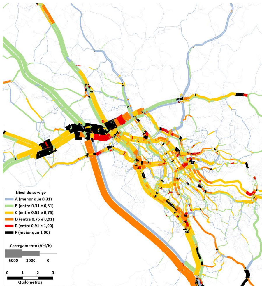
Figura 127 – Nível de Serviço – Ano 2030 – “Nada a Fazer”
