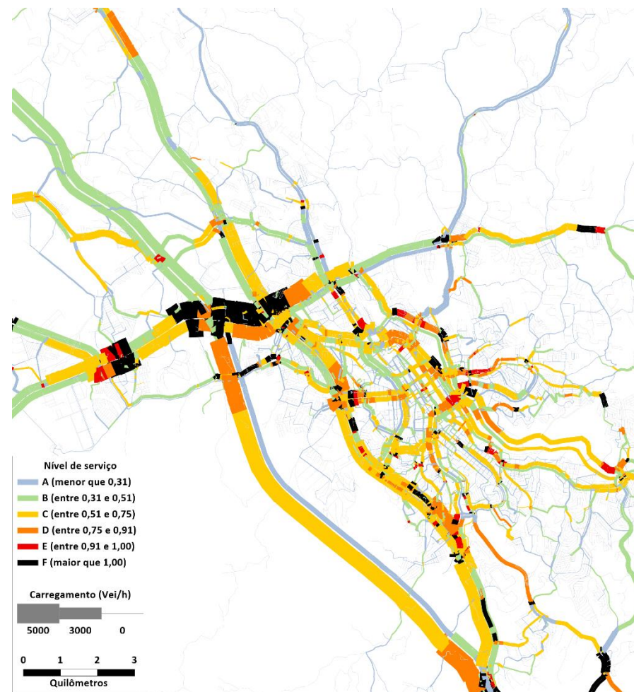
Figura 124 - Nível de Serviço – Ano 2024 – “Faseado”
