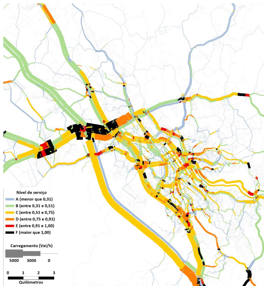
Figura 123 – Nível de Serviço – Ano 2024 – “Nada a Fazer”
