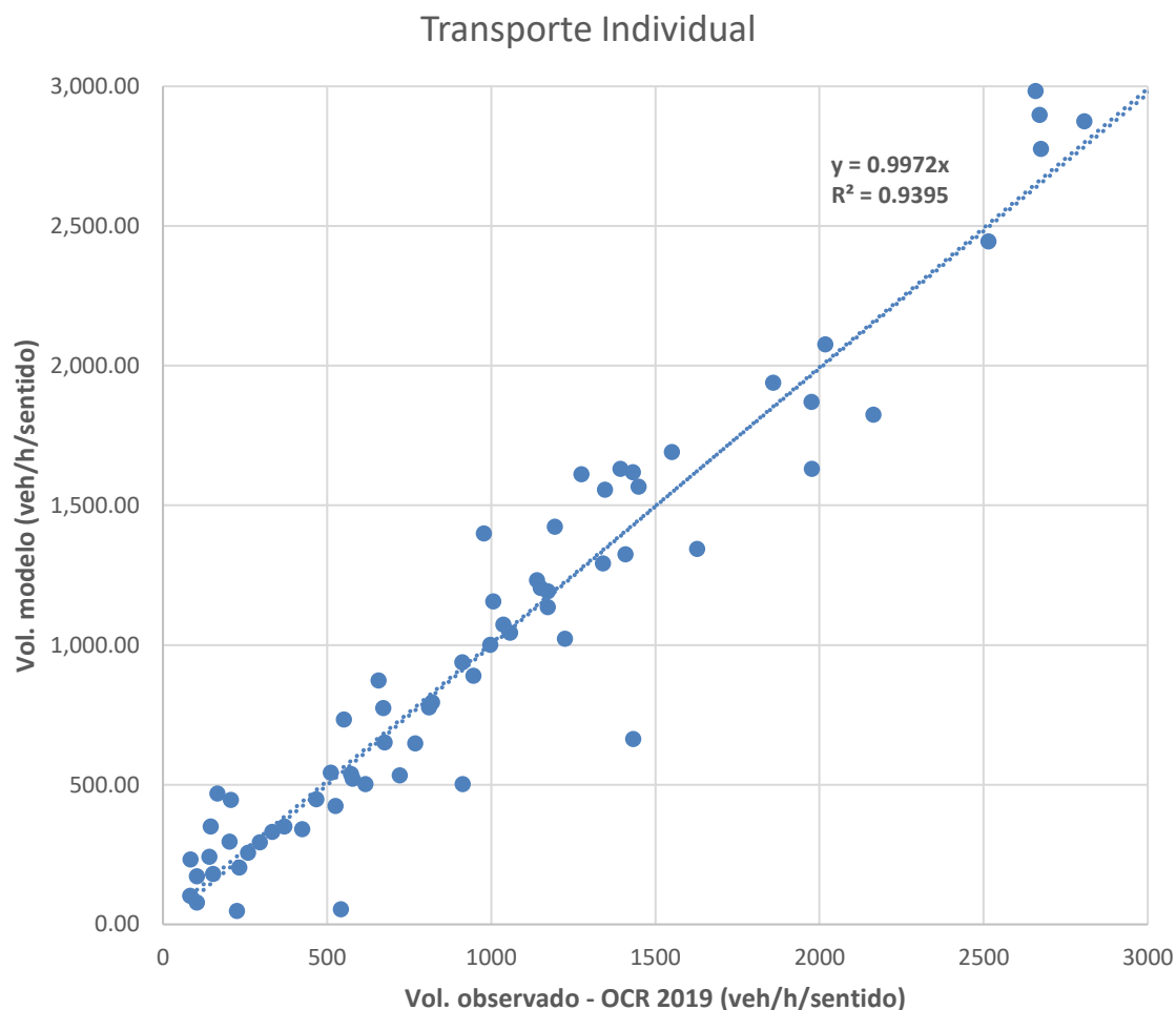
Figura 28: Comparação fluxos observados (Vol OCR 2019) e simulado (Vol Modelo) nos pontos de contagem
