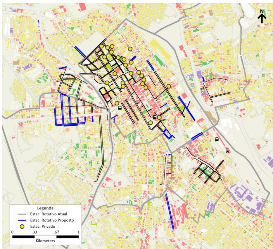
Figura 117 – Localização dos bolsões de estacionamento – Região Central
