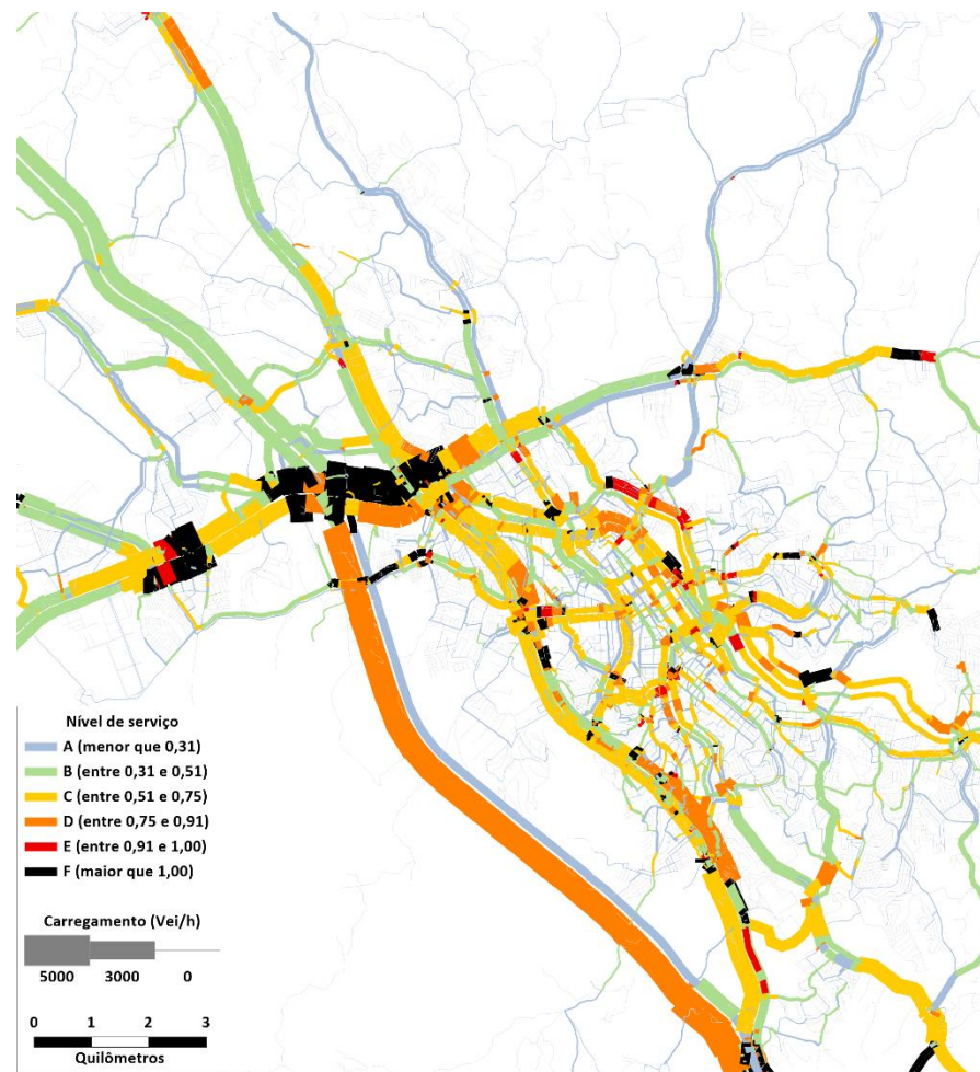
Figura 128 - Nível de Serviço – Ano 2030 – “Faseado”
