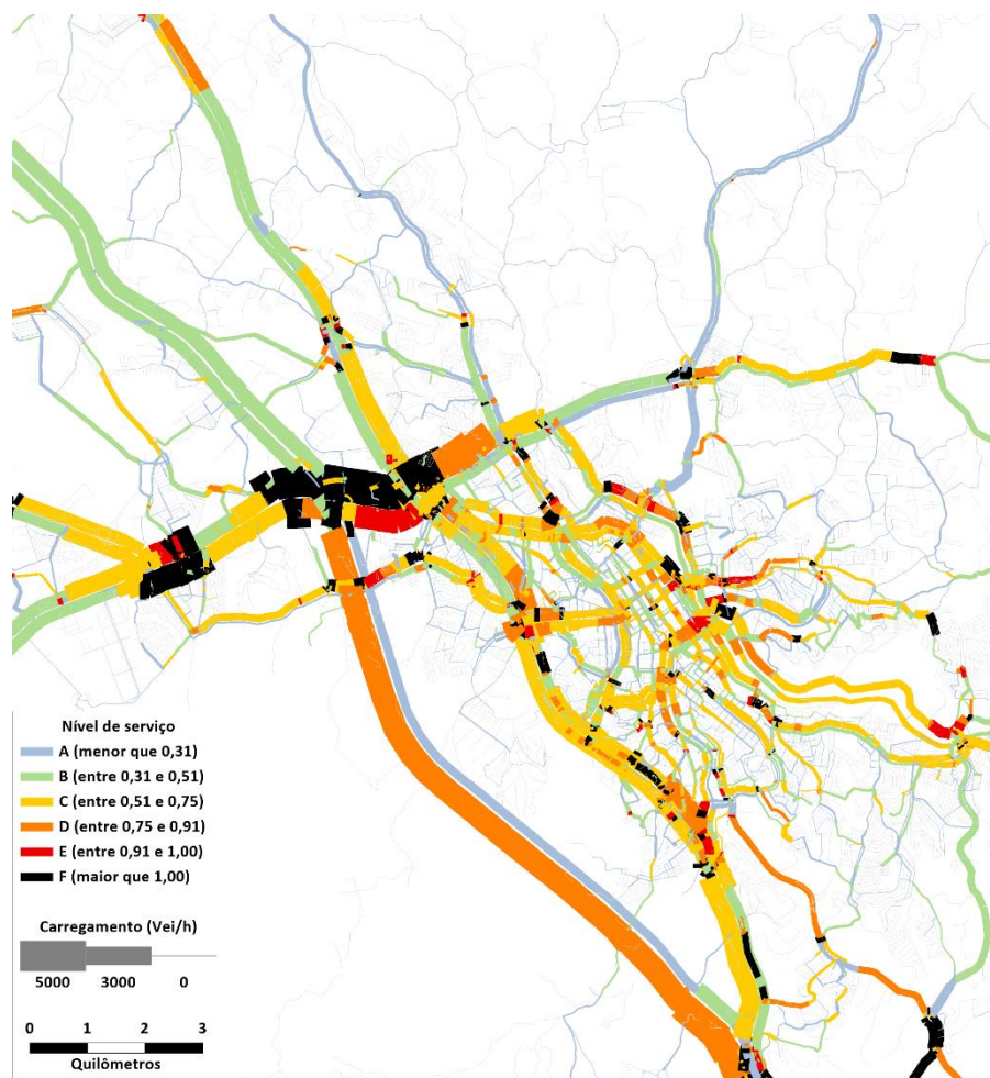
Figura 125 – Nível de Serviço – Ano 2027 – “Nada a Fazer”
