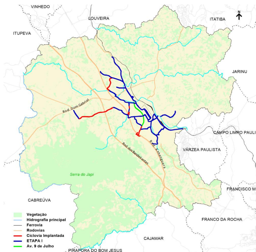
Figura 106: Etapa I – Rede proposta
