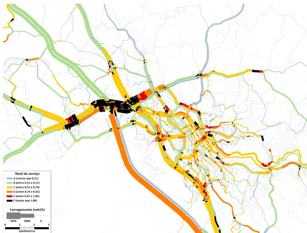
Figura 122 – Nível de Serviço – Ano Base
